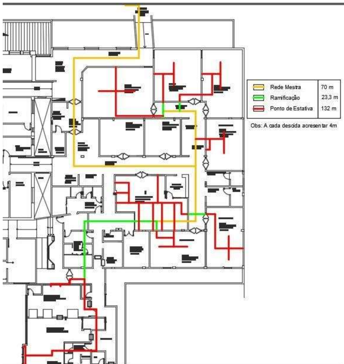
Imagem 01: Croqui com rede dos gases. (Autor)
