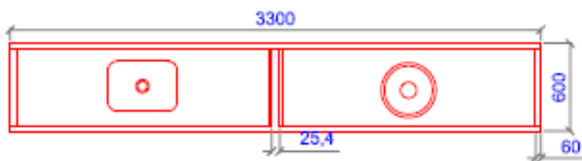
Vista Superior
