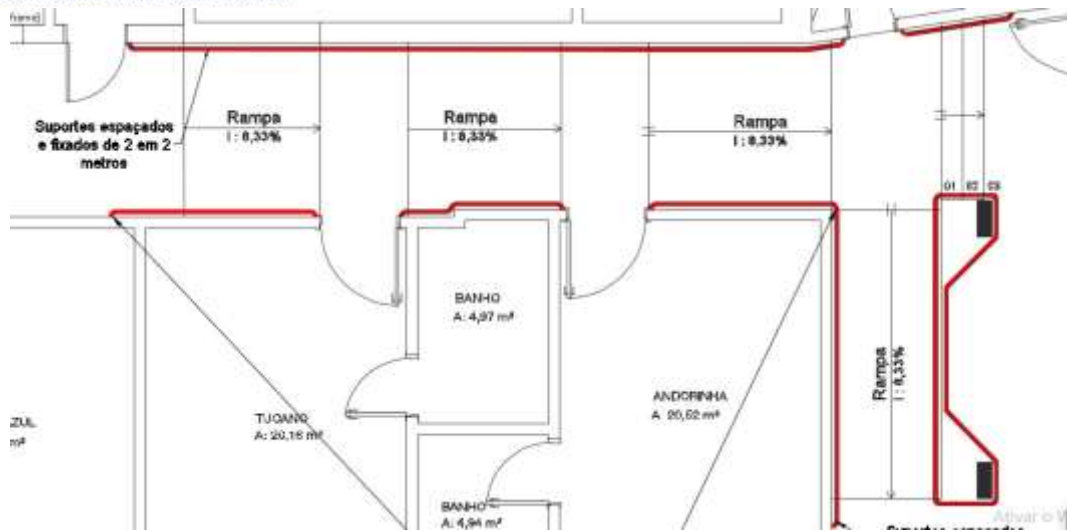
Imagem 01: Detalhe de corrimões, ver mais na prancha em anexo.
