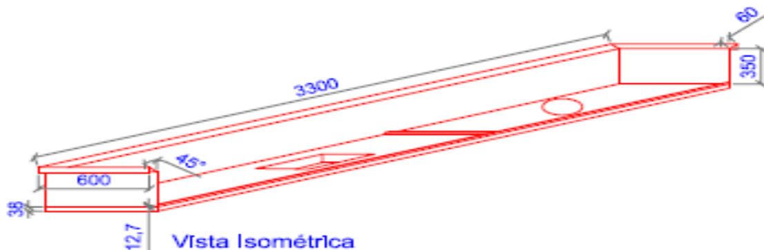
TAMPO HUST - 5 medidas em mm
